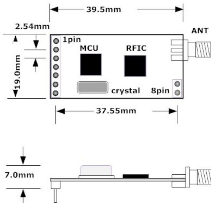
图一 产品尺寸图
